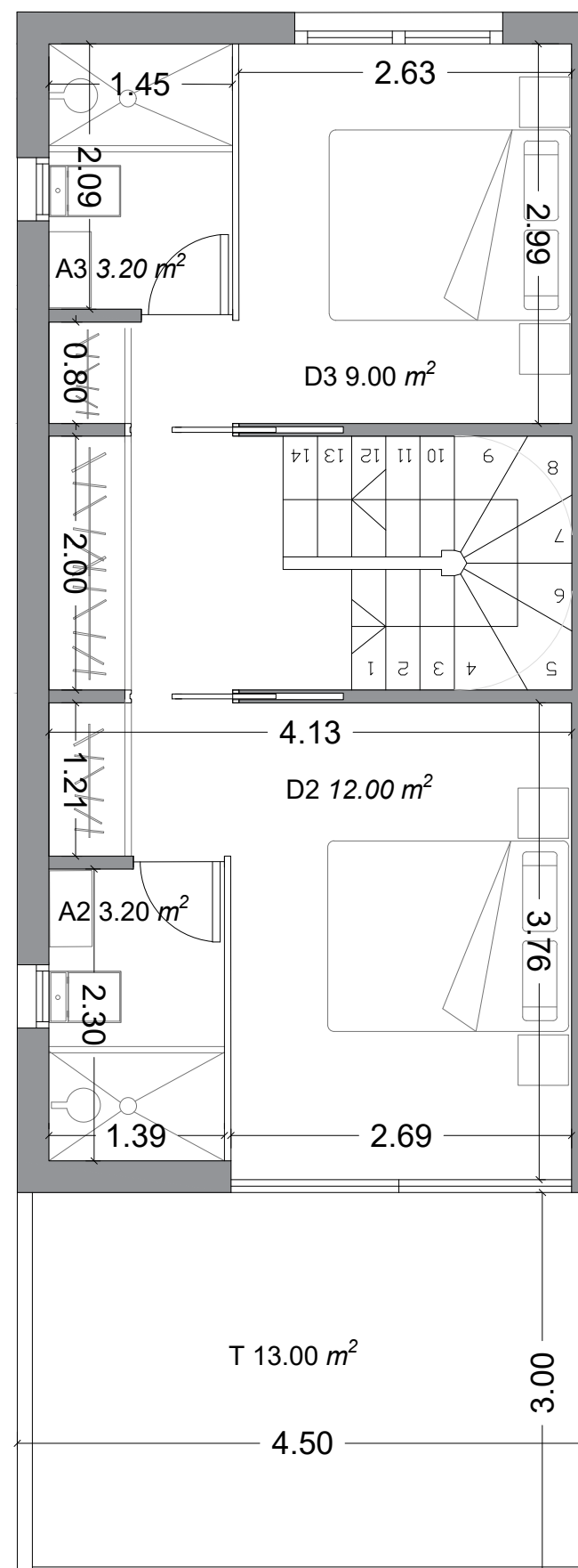
PLANTA PRIMERA
