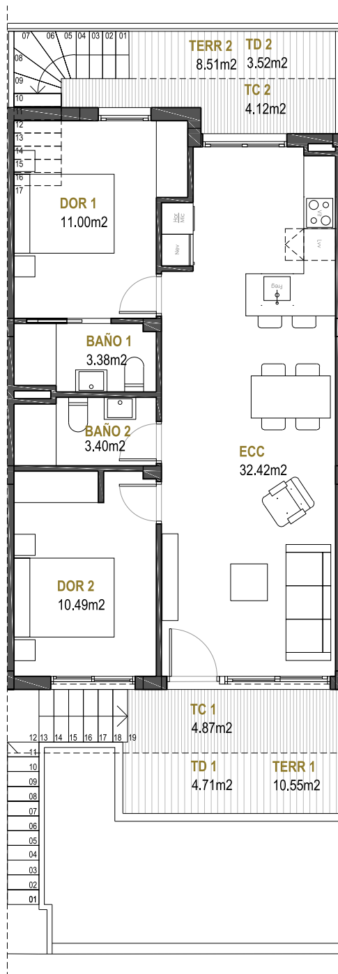
PLANTA PRIMERA
