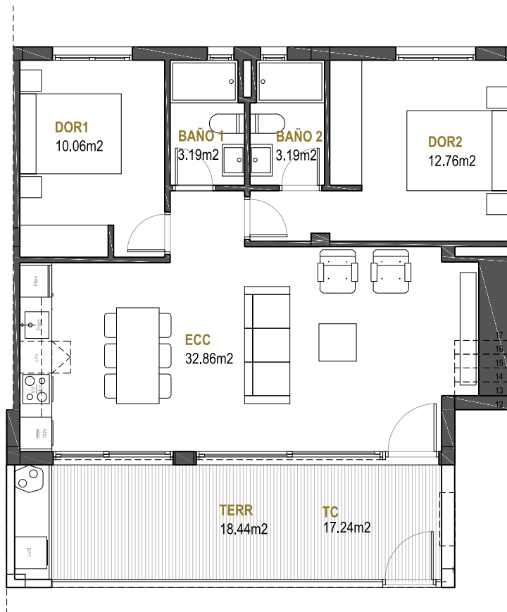
PLANTA BAJA
