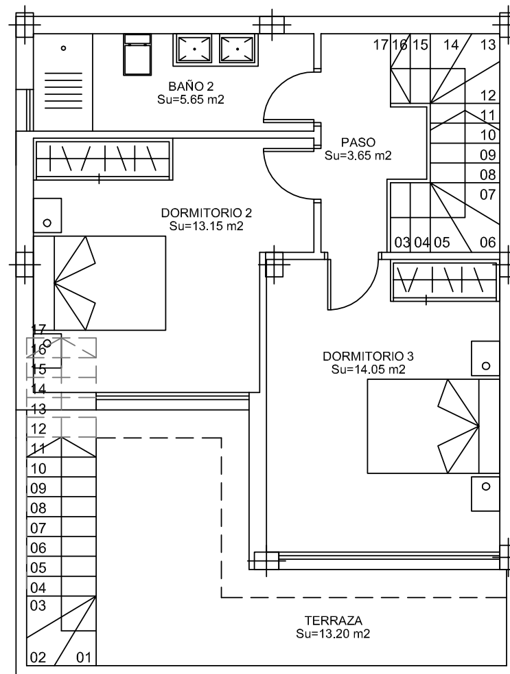
PLANTA PRIMERA
